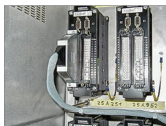
DIN Connector
