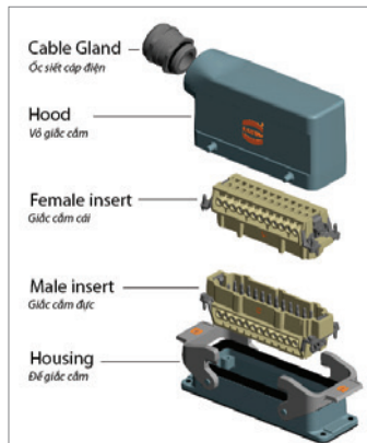
Han Connector
